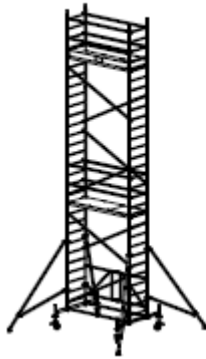
Art. nr 920065P Wys. robocza: 8,8m Wys. ruszt.: 7,8m Wys. do pom.: 6,8m
