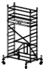
Art. nr 920027P Wys. robocza: 4,8m Wys. ruszt.: 3,8m Wys. do pom.: 2,8m
