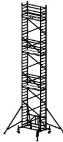
Art nr 920096P Wys. robocza: 11,8m Wys. ruszt.: 10,8m Wys. do pom.: 9,8m
