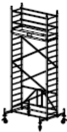
Art nr 920034P Wys. robocza: 5,8m Wys. ruszt.: 4,8m Wys. do pom.: 3,8m
