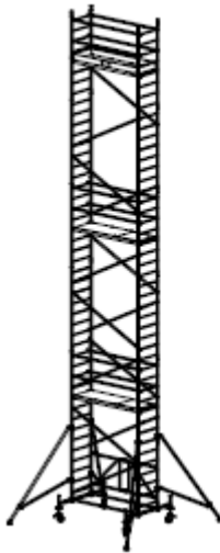
Art nr 920102 Wys. robocza: 12,8m Wys. ruszt.: 11,8m Wys. do pom.: 10,8m
