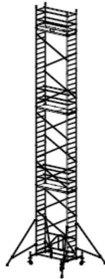
Art nr 920119 Wys. robocza: 13,8m Wys. ruszt.: 12,8m Wys. do pom.: 11,8m
