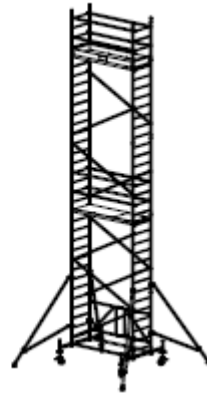
Art. nr 920072P Wys. robocza: 9,8m Wys. ruszt.: 8,8m Wys. do pom.: 7,8m
